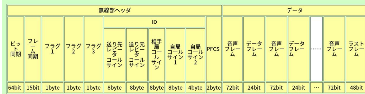
図1. D-STARパケット <JARL D-STARのデジタル音声通信>より
